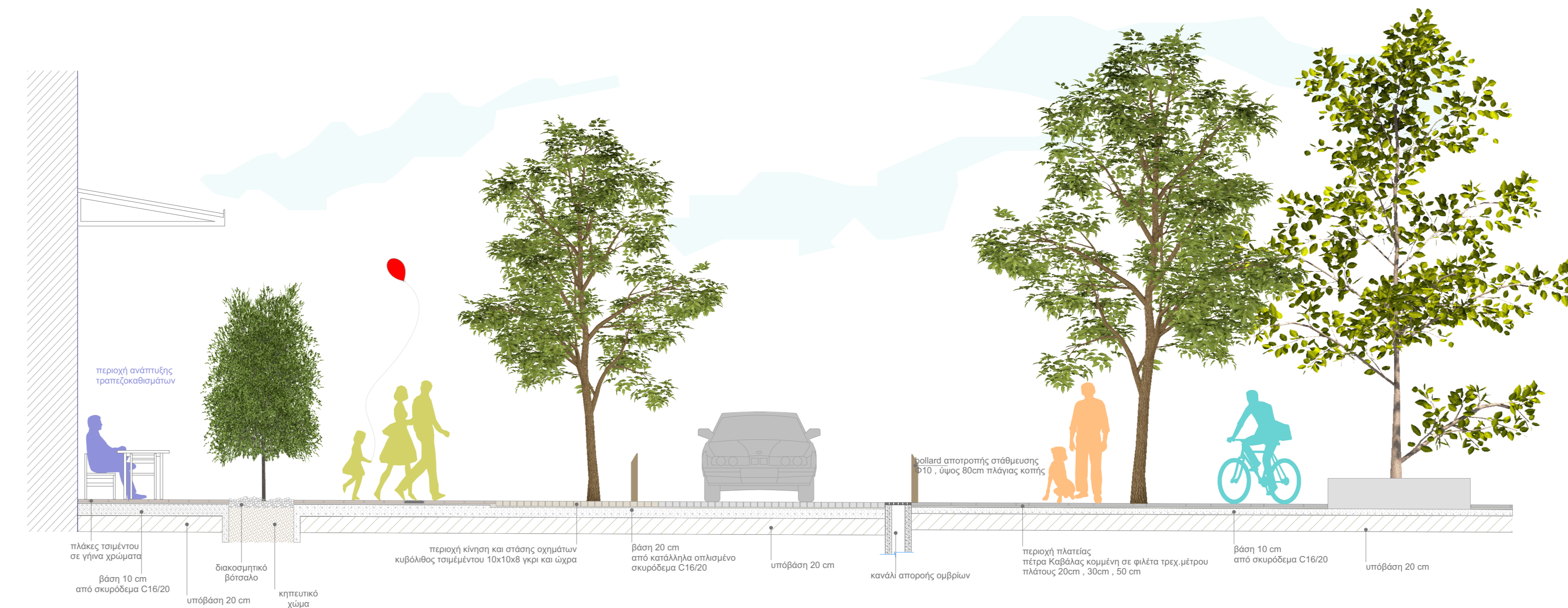
ΤΟΜΗ Τ1 κλιμ. 1:50
