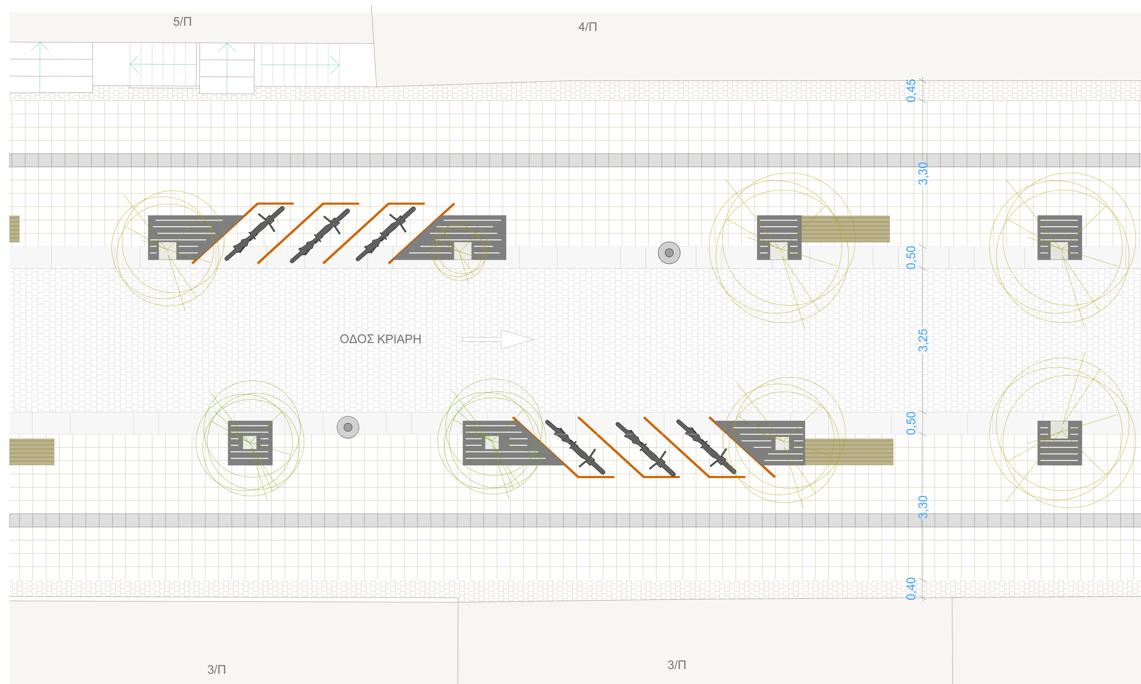
ΛΕΠΤΟΜΕΡΕΙΑ ΟΔΟΣ ΚΡΙΑΡΗ κλιμ. 1:50
